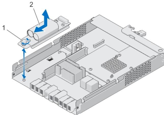
Abbildung 22. Entfernen und Installieren des RAID-Controller-Modul-Akkusicherungsmoduls
