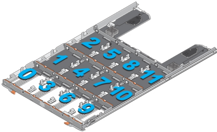
Abbildung 14. Steckplatznummerierung in der Laufwerksschublade
